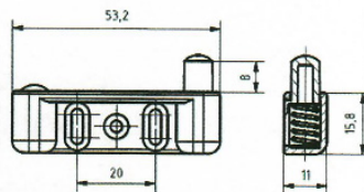
Gedämpfter Schließwinkel 0°-10° 434690
