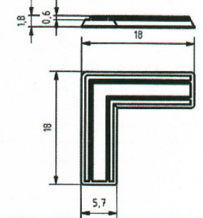
Schweißwinkel 404012
