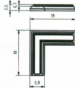
Schweißwinkel 404032
